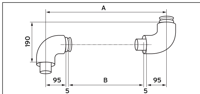
Рис. 6.80 Монтаж колен 87°
