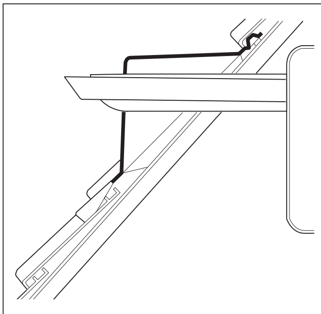
Рис. 5.10 Пример монтажа горизонтального кровельного ввода (слуховое окно)
