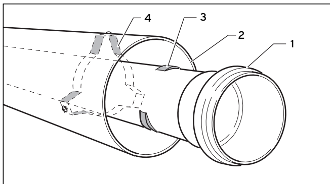
Рис. 6.78 Ослабление трубы газоотвода
