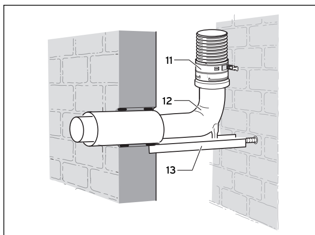
Рис. 5.53 Концентрическое подсоединение к гибкому выпускному газопроводу
