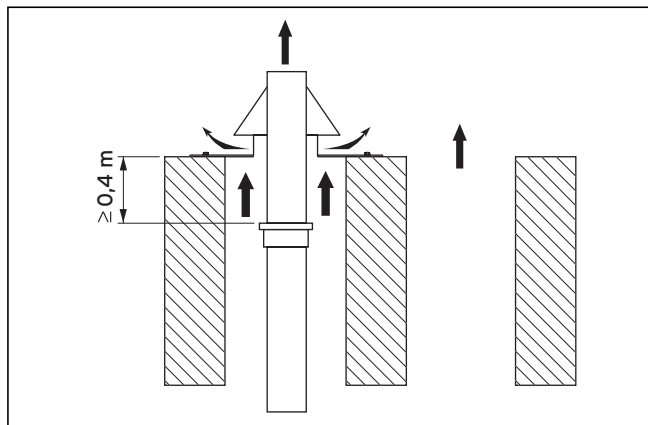
Рис. 5.68 Высота дымовой трубы над выпускным газопроводом из ПП с устьем из нержавеющей стали - с забором воздуха из помещения
