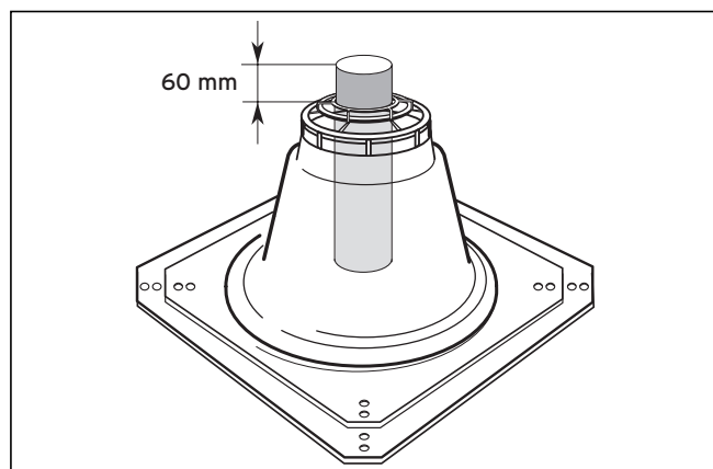
Рис. 6.73 Длина верхней трубы газопровода
