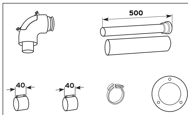
Рис. 5.31 Объем поставки арт. № 303 923
