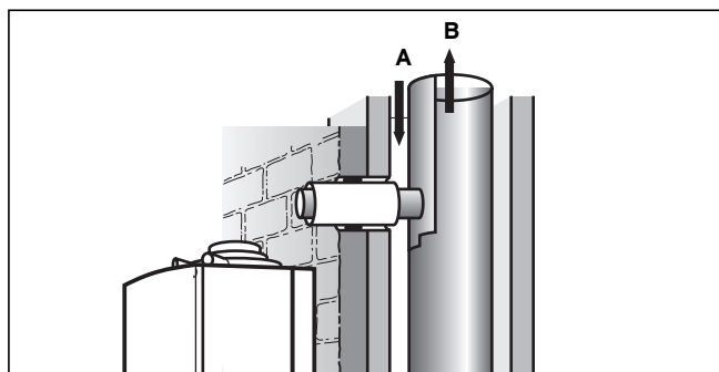
Рис. 5.33 Укорачивание длины трубы газопровода и установка трубы воздухопровода
