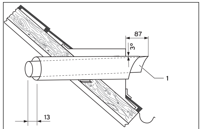
Рис. 5.26 Вмонтаживание горизонтального кровельного ввода
