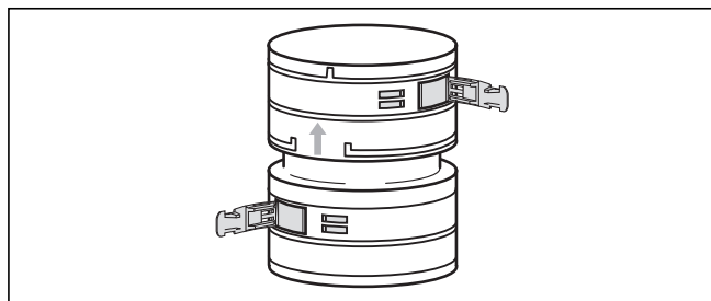
Рис. 6.50 Соединительный элемент
