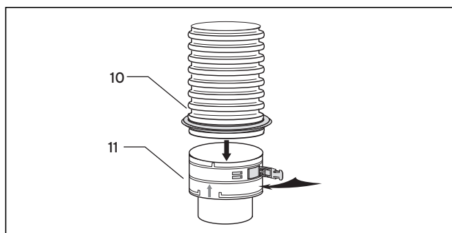
Рис. 5.51 Вставной элемент с гибким выпускным газопроводом
