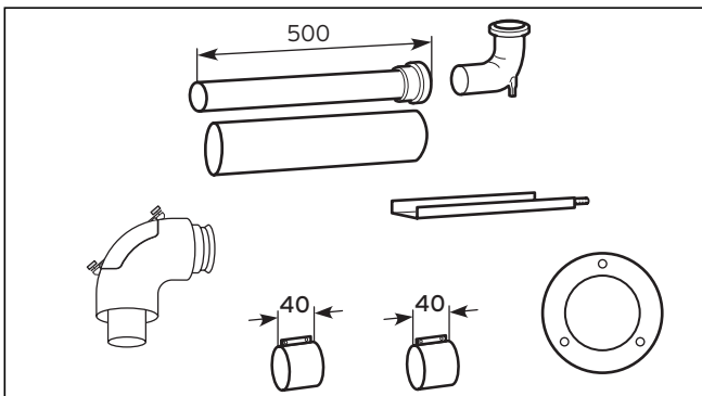
Рис. 5.38 Объем поставки
