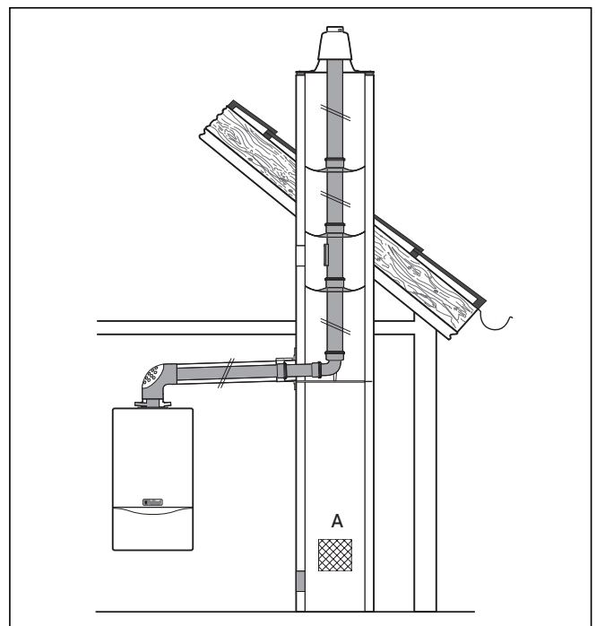
Рис. 5.40 Пример монтажа с забором воздуха из помещения
