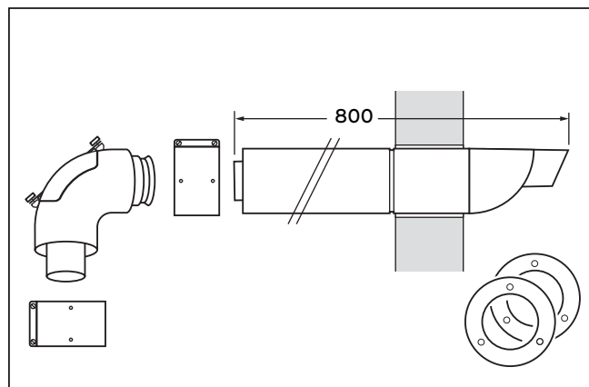
Рис. 5.6 Объем поставки арт. № 303 922
