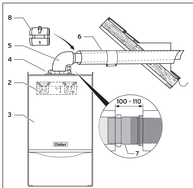
Рис. 5.30 Удаленная установка
