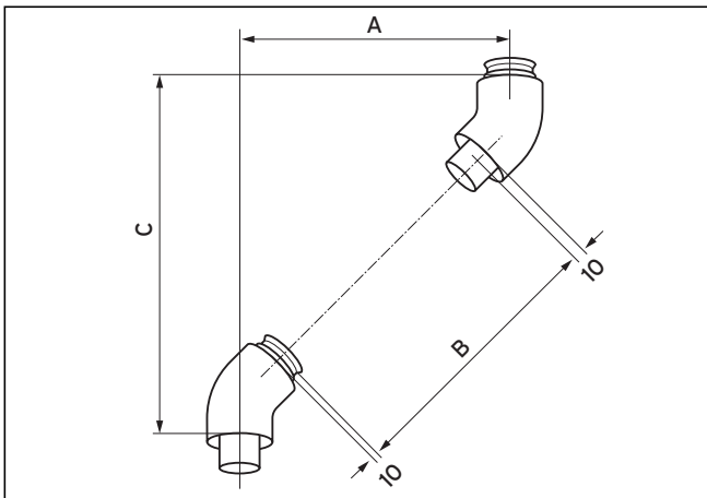
Рис. 5.74 Монтаж колен 45°
