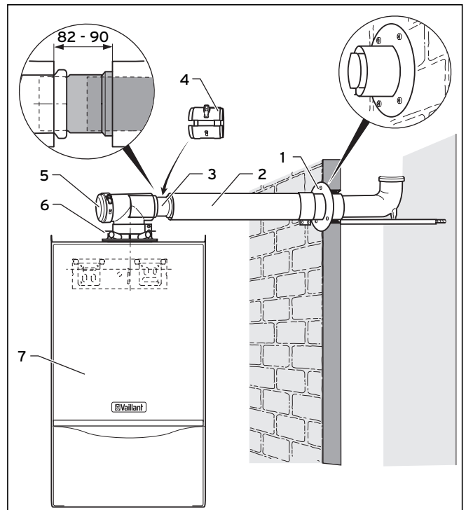
Рис. 6.26 Монтаж горизонтального участка
