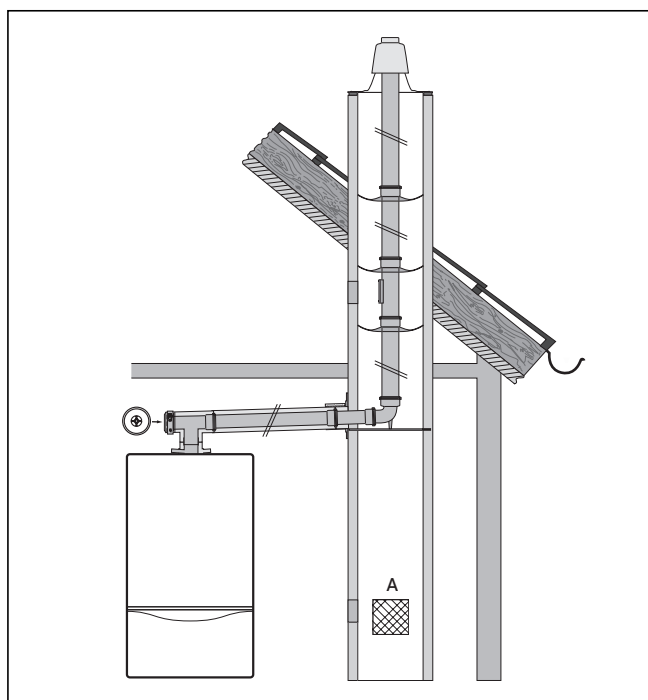
Рис. 6.19 Пример монтажа с забором воздуха из помещения
