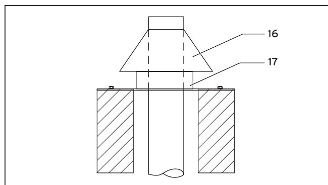
Рис. 6.49 Монтаж шахтного перекрытия
