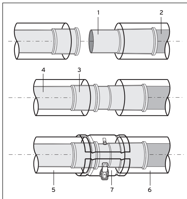
Рис. 6.1 Монтаж разделителя
