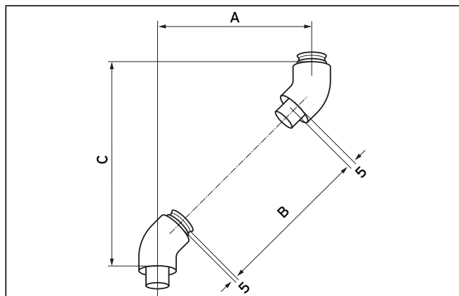
Рис. 6.81 Монтаж колен 45°
