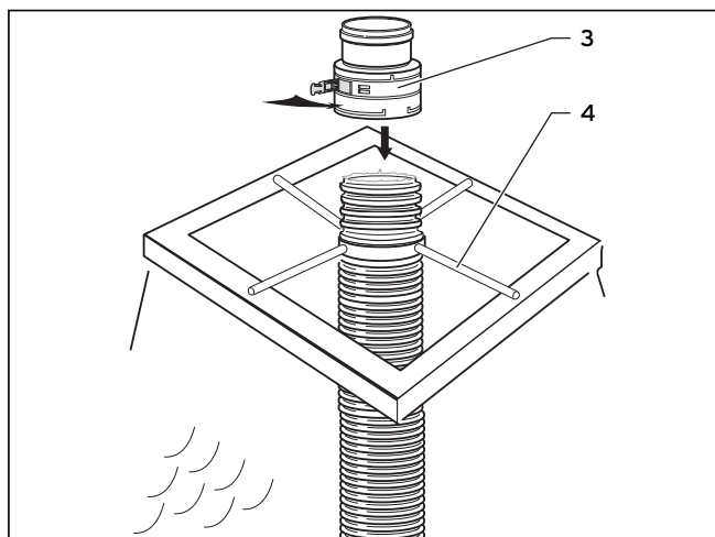
Рис. 5.58 Монтаж соединительной детали
