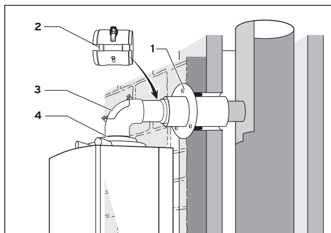
Рис. 5.34 Монтаж прибора
