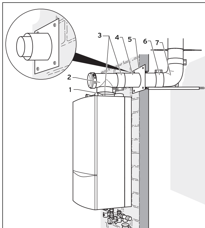
Рис. 6.76 Прямая установка
