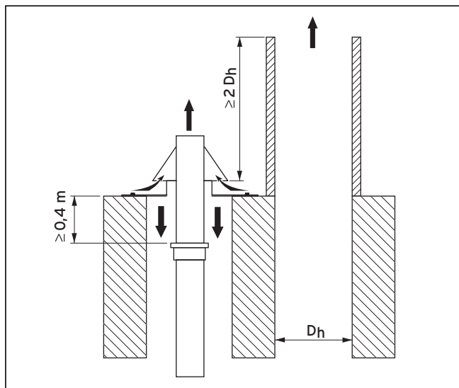
Рис. 5.67 Высота дымовой трубы над выпускным газопроводом из ПП с устьем из нержавеющей стали - с забором воздуха не из помещения
