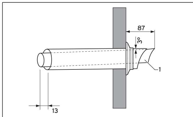
Рис. 5.27 Монтаж горизонтального ввода через стену
