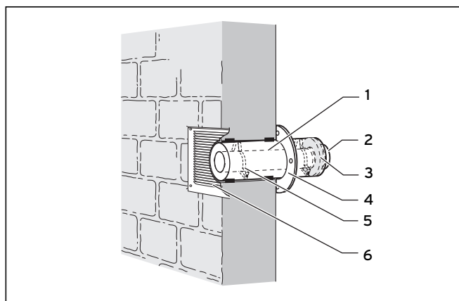
Рис. 6.33 Монтаж воздухозаборника
