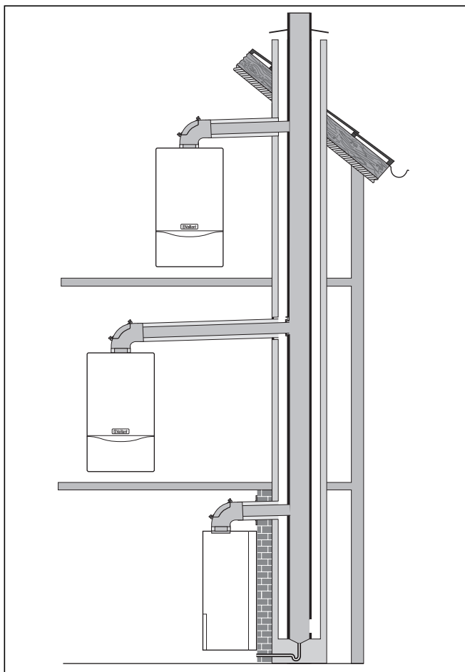
Рис. 5.32 Пример монтажа:
