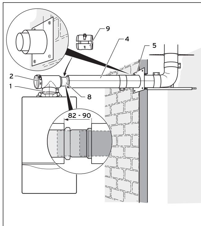
Рис. 6.77 Удаленная установка
