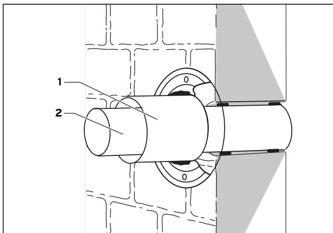
Рис. 5.36 Монтаж подсоединения
