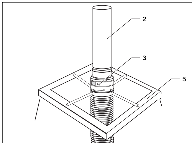
Рис. 6.61 Монтаж трубы устья
