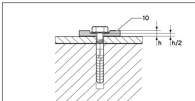
Рис. 6.75 Крепление гибкими подкладными шайбами
