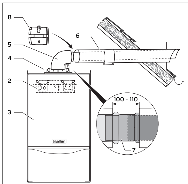
Рис. 5.21 Удаленная установка
