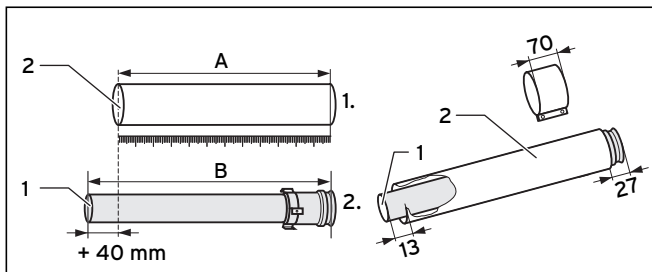
Рис. 5.72 Укорачивание труб
