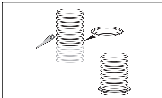
Рис. 5.50 Укорачивание гибкого выпускного газопровода и монтаж уплотнения
