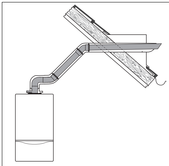
Рис. 5.9 Пример монтажа горизонтального ввода через стену/ кровельного ввода
