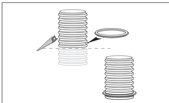
Рис. 6.54 Укорачивание гибкого выпускного газопровода и монтаж уплотнения
