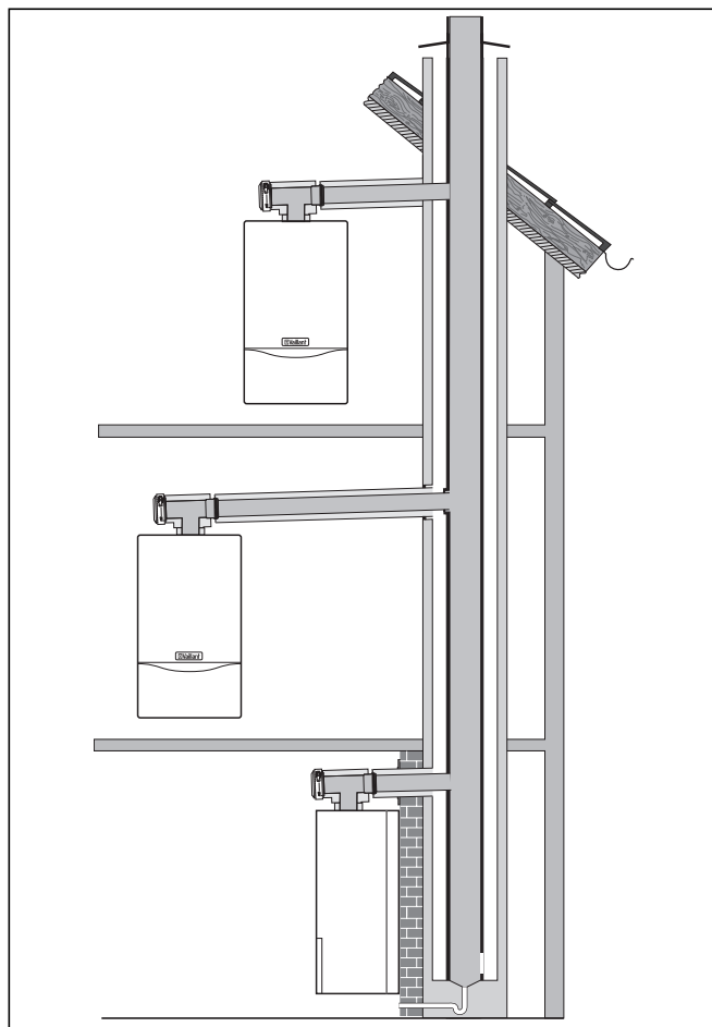
Рис. 6.11 Пример монтажа:
