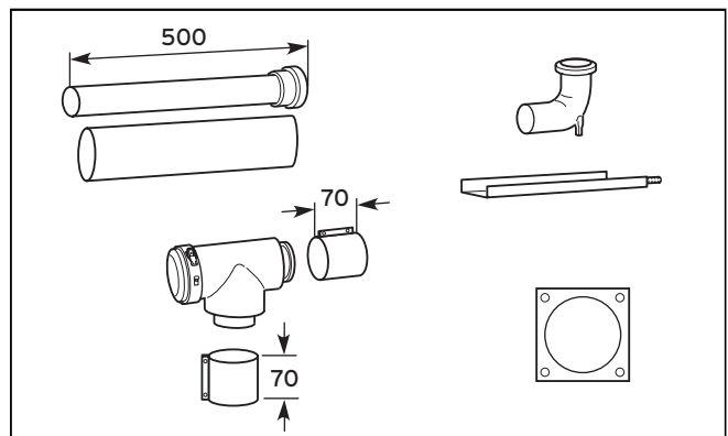
Рис. 6.17 Объем поставки
