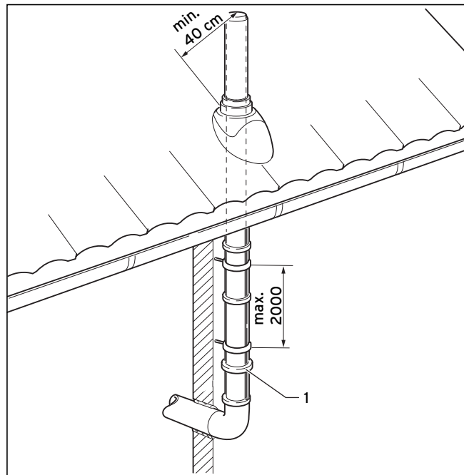
Рис. 6.70 Монтаж выпускного газопровода на наружном фасаде
