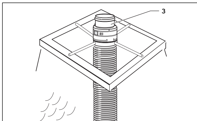
Рис. 5.59 Соединительная деталь с гибким выпускным газопроводом
